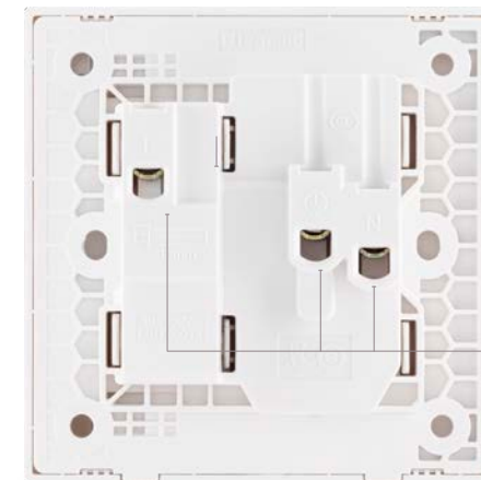
带单控开关五孔插座3个接线端子， 免跨接线、安装便捷，安全跃级。
