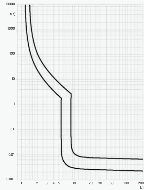
■ 脱扣特性C曲线
