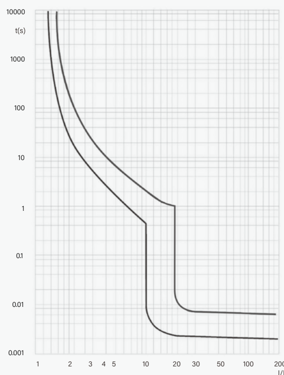
■ 脱扣特性D曲线
