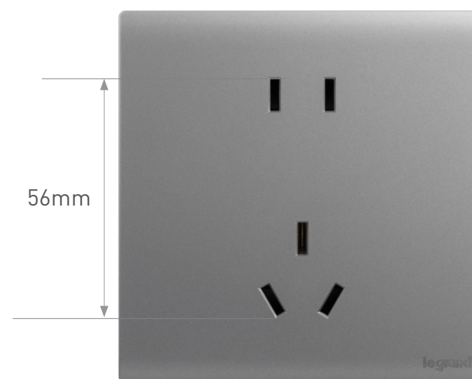
大间距56mm 满足不同厨电的同时用电需求。
