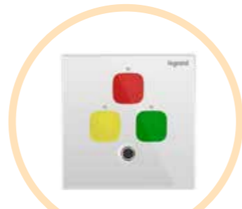
有线多功能坠式求助器 型号：NE1014231-01C-W
