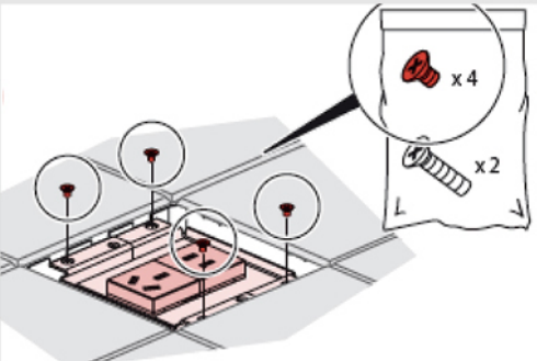
混凝土地板上（配预埋盒）
