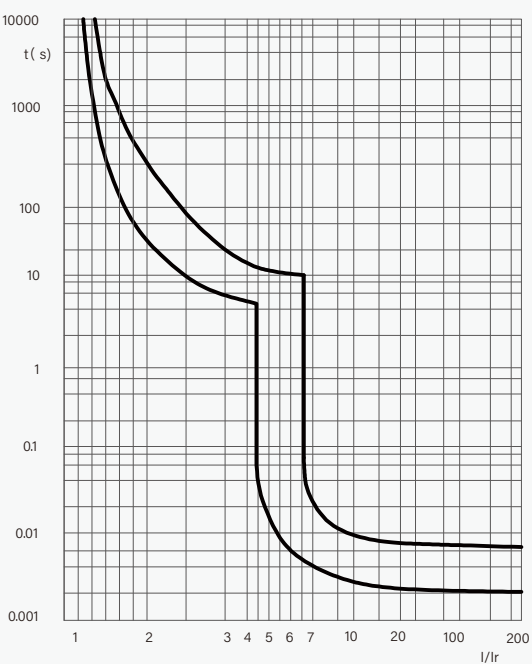
B 曲线: I_i=5.5I_n\pm20\%
