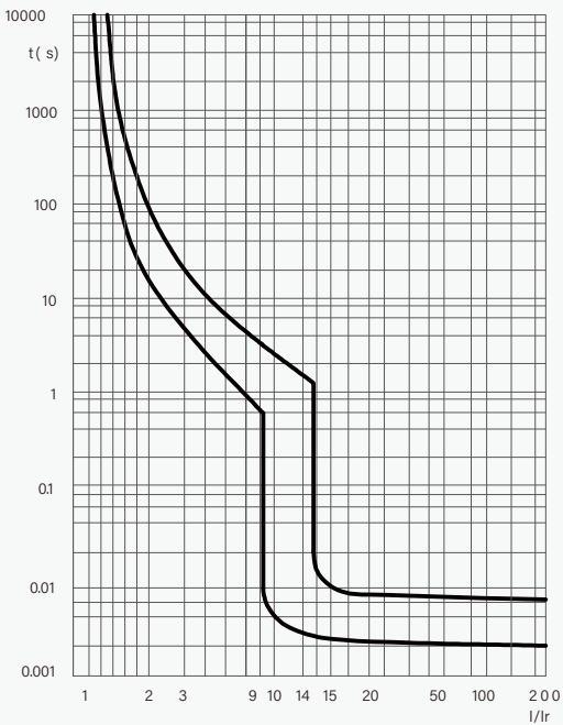
D 曲线: I_i=12I_n\pm20\%
