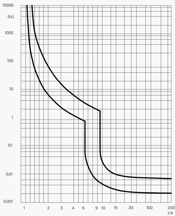
C曲线: I_i=8I_n\pm20\%
