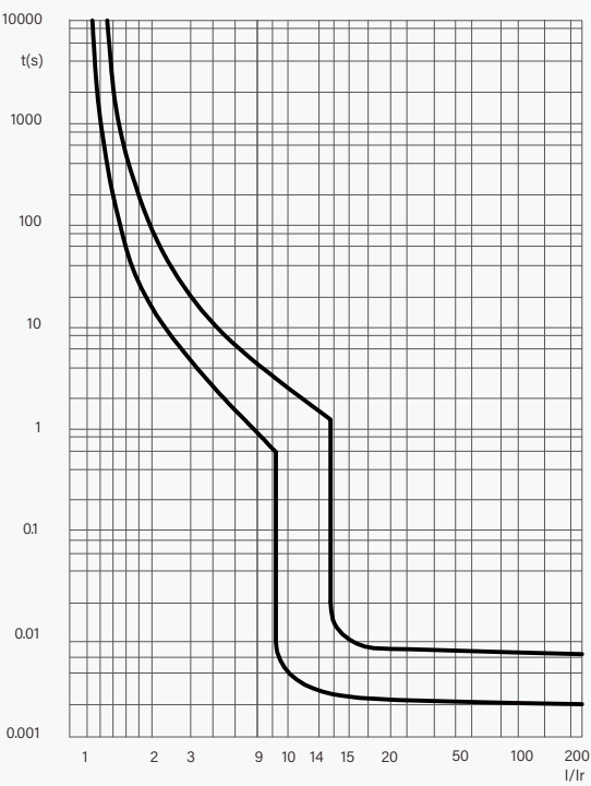
D曲线: I_i=12I_n\pm20\%
