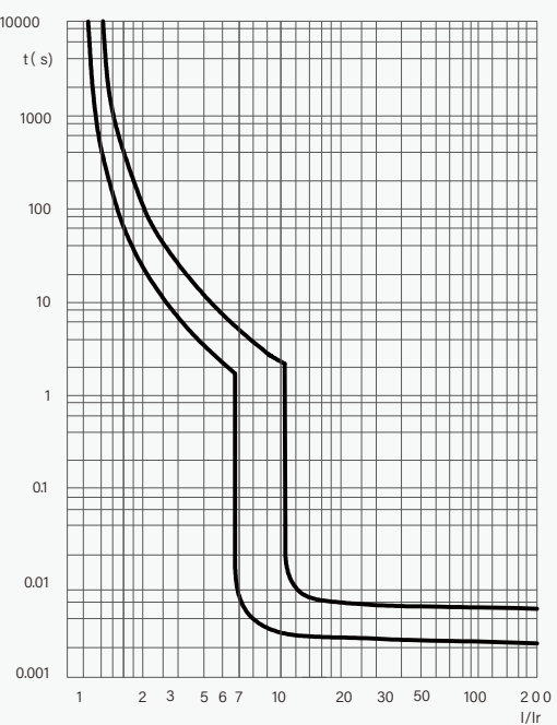
C 曲线: I_i=8.5I_n\pm20\%
