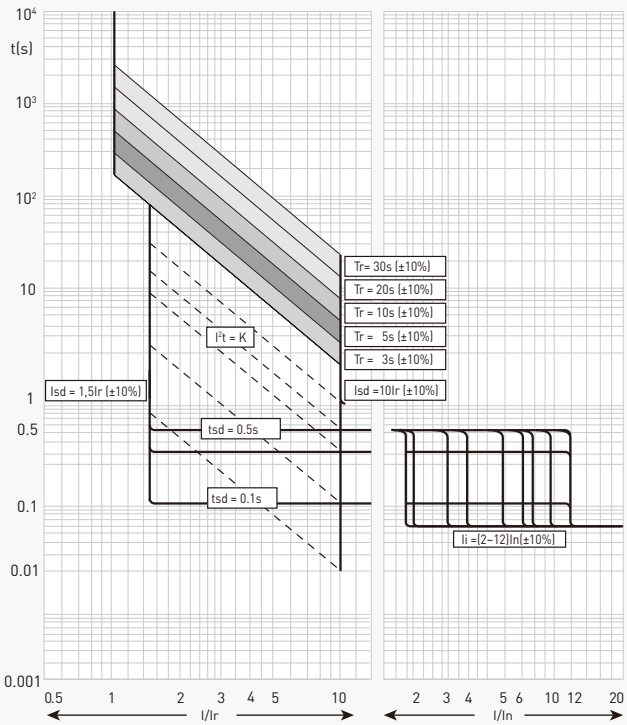
400/630/800电子式脱扣曲线
