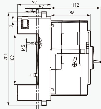
板后接线
