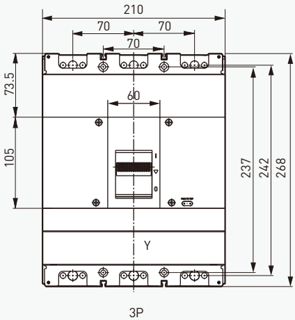
■ TMX 800固定式 板前接线
