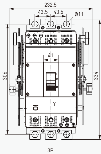
■ TMX 400/630抽出式 板前接线
