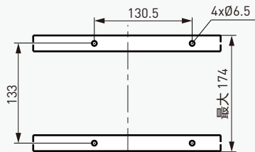
板后导轨安装 4P
