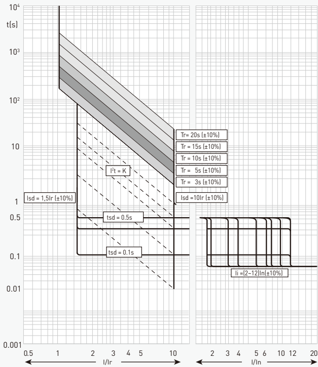
250 HP 电子式脱扣曲线
