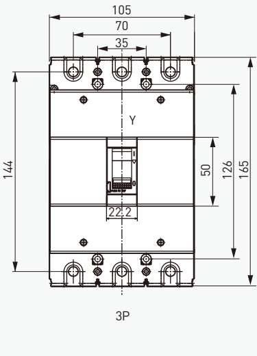
■ TMX 250 HP 固定式 板前接线
