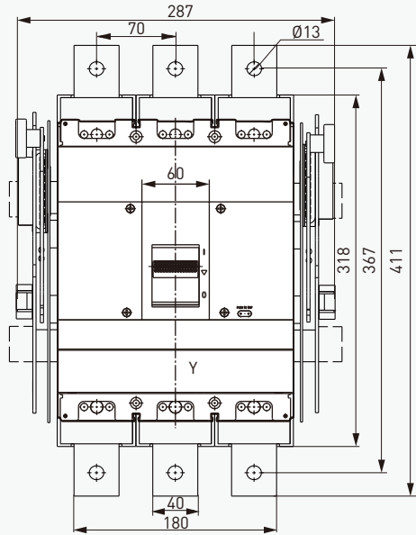
■ TMX 800抽出式 板前/板后接线
