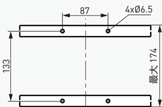
板后导轨安装 3P
