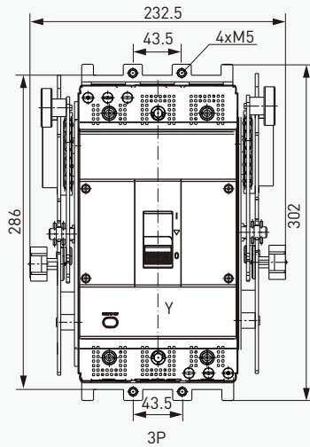
■ TMX 400/630抽出式 板后接线
