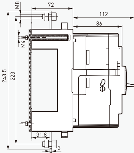
板后接线
