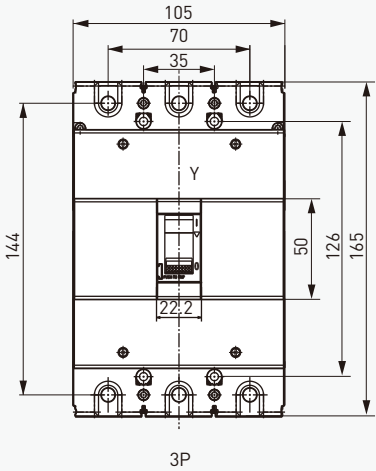
■ TMX 250固定式 板前接线
