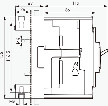
板后接线
