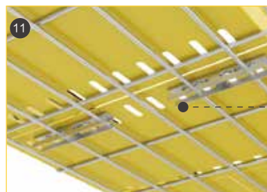
底部连接件：与专用螺钉配套使用，将直线段底部固定在网格式桥架上，确保直线段定位准确，安装牢固。
