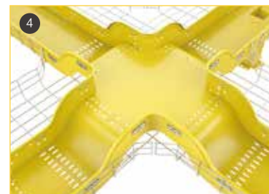
四通转接：用来提供直线段的分支和变径。
