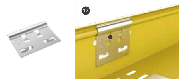
侧部快速连接板：直线段侧部无螺丝快速连接。
