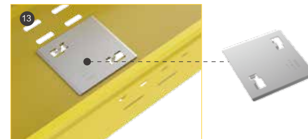
底部快速连接板：直线段底部无螺丝快速连接。
