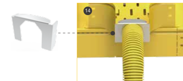
波纹管固定板：将波纹管快速和光纤槽固定。
