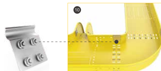
侧面连接板：OFT部件间侧部连接。
