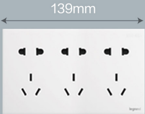
十五孔插座
