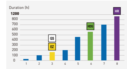
盐雾试验(中性盐雾)是电缆桥架最常用和公认的试验，参考IEC 61537
