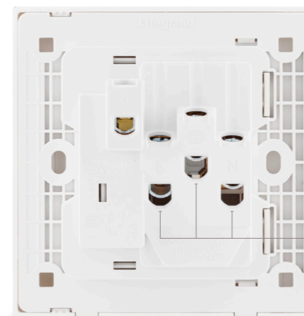
带开关五孔插座4个接线端子 免跨接线、可接负载灯
