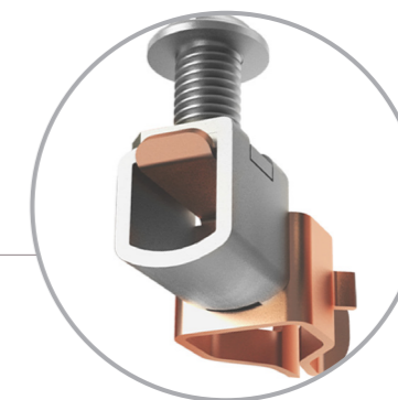
加大鞍形接线端子 接线安装更方便
